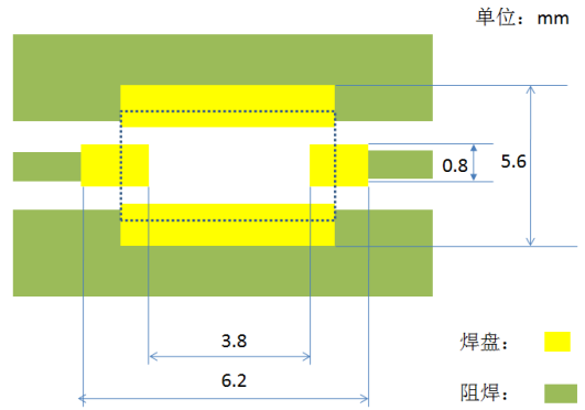
PCB推荐焊盘
